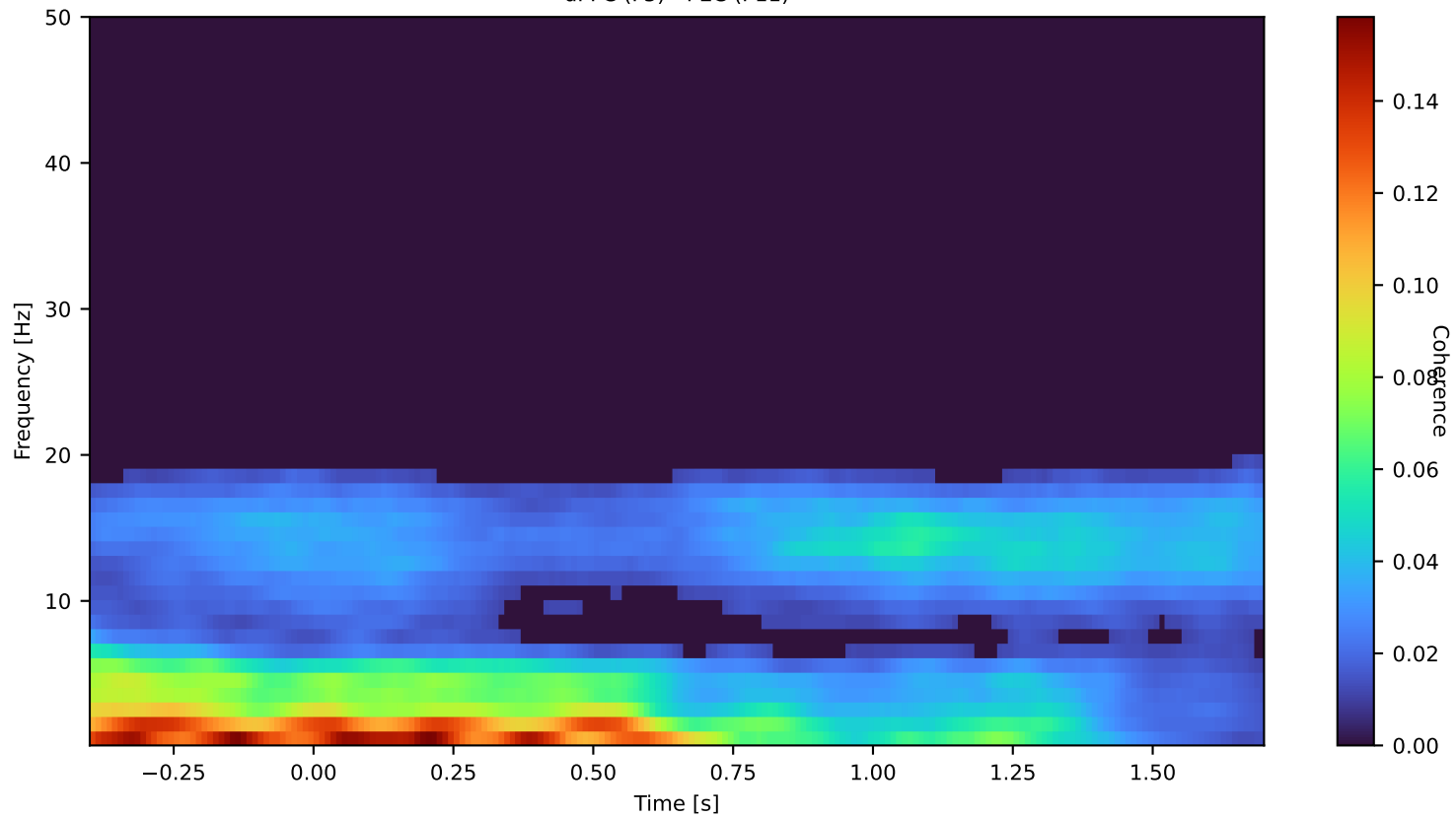
dPFC (F5) - PEC (P11)
